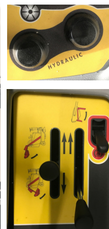
Bedien voor het heffen en ledigen van de vuilbak altijd de 2 ronde knoppen van de hydrauliek. Gebruik daarna de hendels voor het heffen of het ledigen van de vuilbak. Leeg deze altijd na gebruik!
