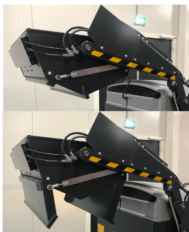
Bedien voor het heffen en ledigen van de vuilbak altijd de 2 ronde knoppen van de hydrauliek. Gebruik daarna de hendels voor het heffen of het ledigen van de vuilbak. Leeg deze altijd na gebruik!
